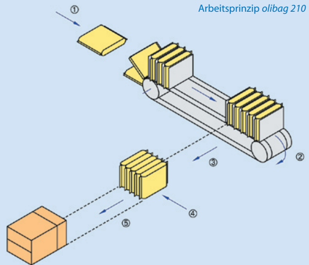
Arbeitsprinzip olibag 210
