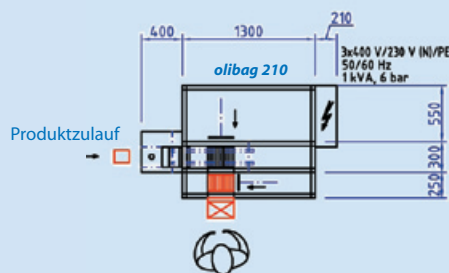
Ansicht Bedienseite
